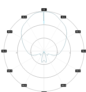
SA M3DBC245-65-9HV H-pol, elev, 5.5GHGz
