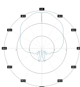
SA M3DBC245-65-9HV V-pol, azimuth, 5.5GHGz
