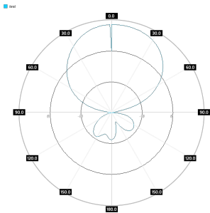
SA M3DBC245-65-9HV H-pol, azimuth, 2.45GHz
