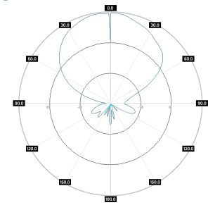
SA M3DBC245-65-9HV H-pol, azimuth, 5.5GHGz
