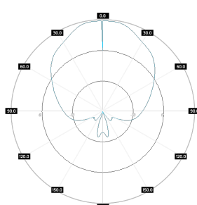
SA M3DBC245-65-9HV H-pol, elev, 5.5GHGz
