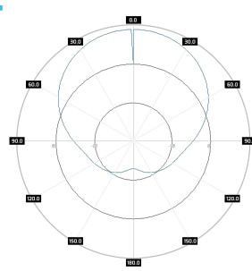
SA M3DBC245-65-9HV V-pol, azimuth, 2.45GHz
