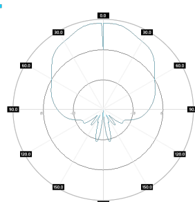
SA M3DBC245-65-9HV V-pol, azimuth, 5.5GHGz
