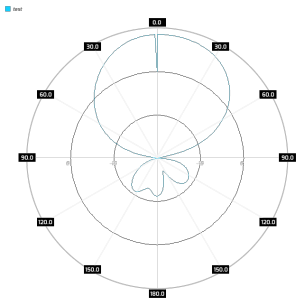
SA M3DBC245-65-9HV H-pol, azimuth, 2.45GHz
