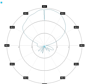
SA M3DBC245-65-9HV V-pol, elev, 5.5GHGz
