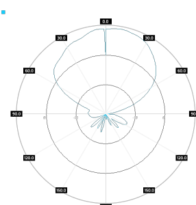
SA M3DBC245-65-9HV V-pol, elev, 5.5GHGz
