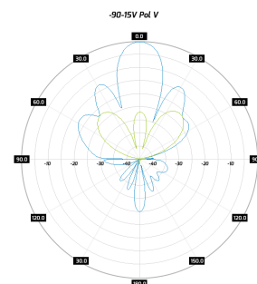
Radiation pattern WiBOX SA 24-90-15V Pol V
