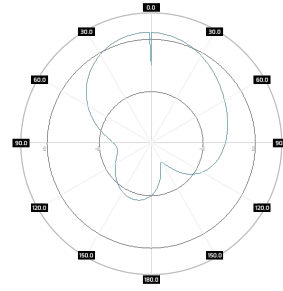
PA MMB0727-8X 800Mhz, port 2, elev.
