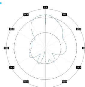
PA MMB0727-8X 2600Mhz, port 2, elev.
