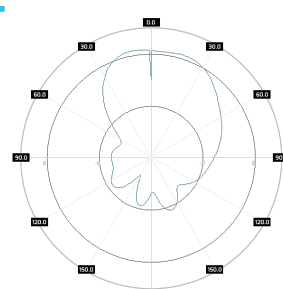
PA MMB0727-8X 2100Mhz, port 2, elev.
