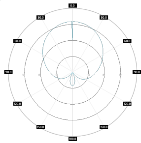
SA M0608-65-12X Port 2, azimuth, 700MHz
