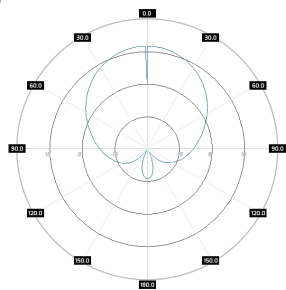
SA M0608-65-12X Port 1, azimuth, 700MHz
