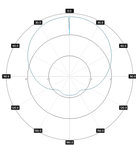
SA M3DBC245-65-9HV H-pol, elev, 2.45GHz
