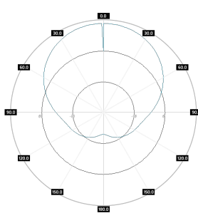
SA M3DBC245-65-9HV V-pol, azimuth, 2.45GHz
