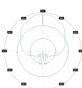
SA M3DBC245-65-9HV V-pol, azimuth, 5.5GHz
