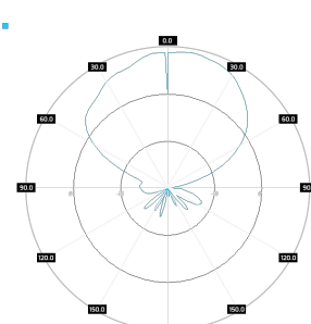
SA M3DBC245-65-9HV V-pol, elev, 5.5GHz
