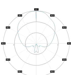
SA M3DBC245-65-9HV H-pol, elev, 5.5GHz
