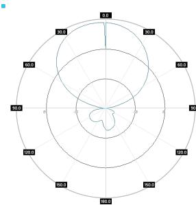
SA M3DBC245-65-9HV V-pol, elev, 2.45GHz
