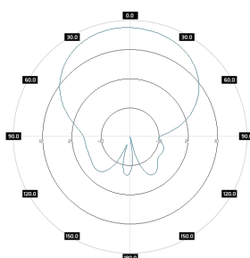
SA M5-90-17HV H-pol, azimuth
