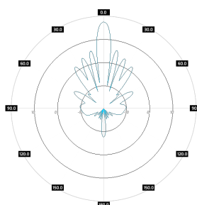
SA M5-90-17HV H-pol, elev.
