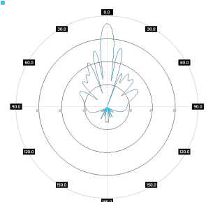
SA M5-90-17HV V-pol, elev.
