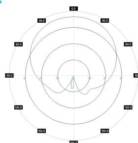
SA M5-90-17HV V-pol, azimuth
