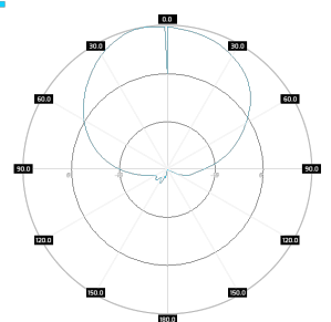
SA M4DBC245-65-9X Slant-pol, elev, 5.5GHz
