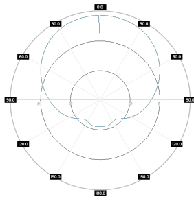
SA M4DBC245-65-9X H-pol, elev, 2.45GHz
