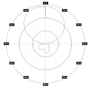
SA M4DBC245-65-9X V-pol, elev, 2.45GHz
