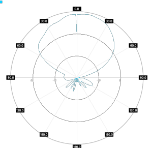
SA M4DBC245-65-9X V-pol, elev, 5.5GHz
