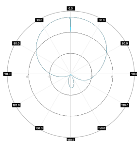
SA M4DBC245-65-9X Slant-pol, elev, 2.45GHz
