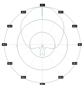
SA M4DBC245-65-9X H-pol, elev, 5.5GHz
