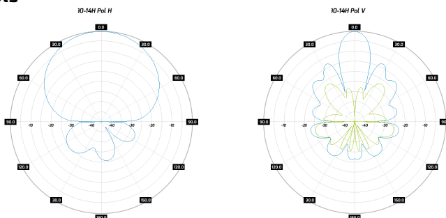
Radiation pattern WiBOX SA 5-90-14H Pol H Radiation pattern WiBOX SA 5-90-14H Pol V
