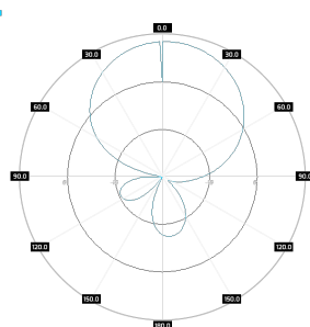
PA 0809-8H Pol H, azimuth
