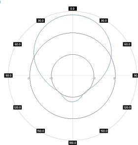
PA 0809-8H Pol H, elev.
