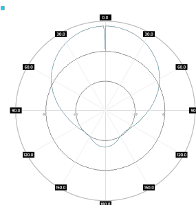
PA 0809-8H Pol H, elev.
