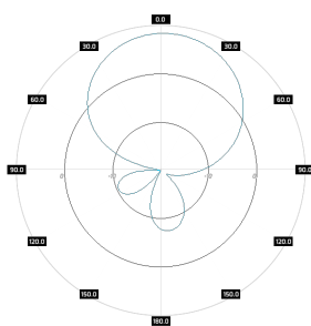
PA 0809-8H Pol H, azimuth
