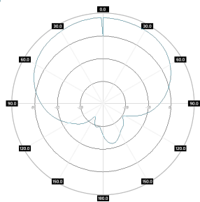
SA MDBC245-120-8V 2.45GHz, azimuth
